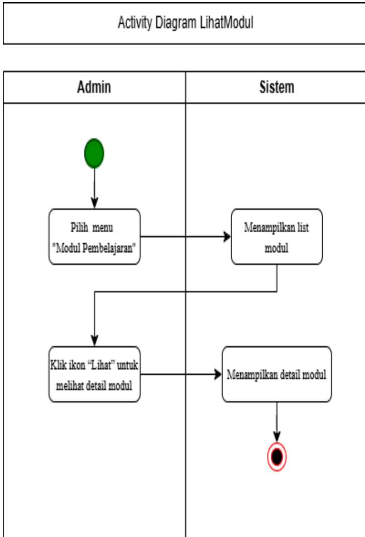
Gambar 6.5 Activity Diagram Melihat Modul Pembelajaran
