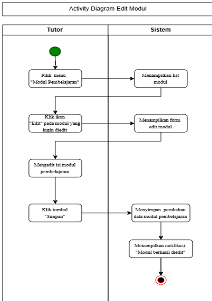
Gambar 6.16 Activity Diagram Tutor Mengedit Modul Pembelajaran
