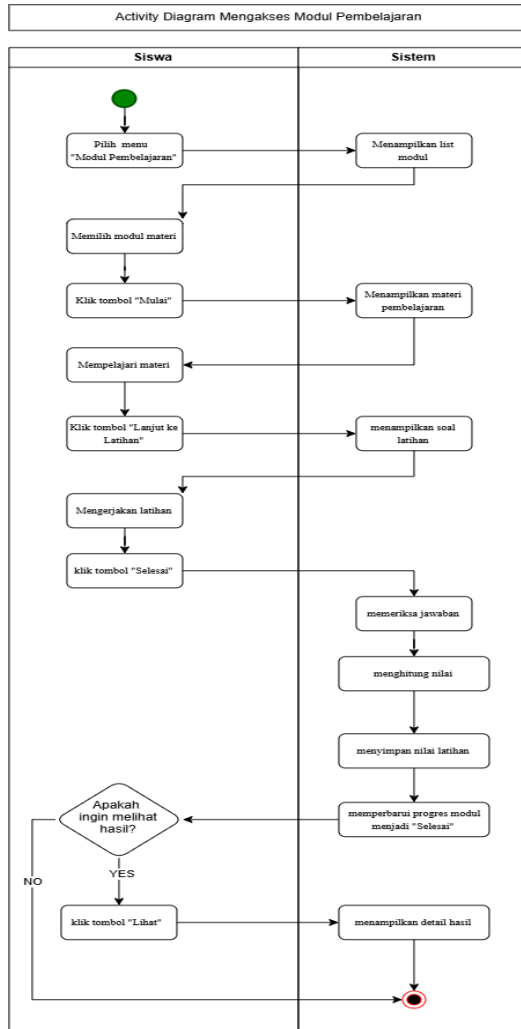
Gambar 6.22 Activity Diagram Siswa Mengakses Modul Pembelajaran
