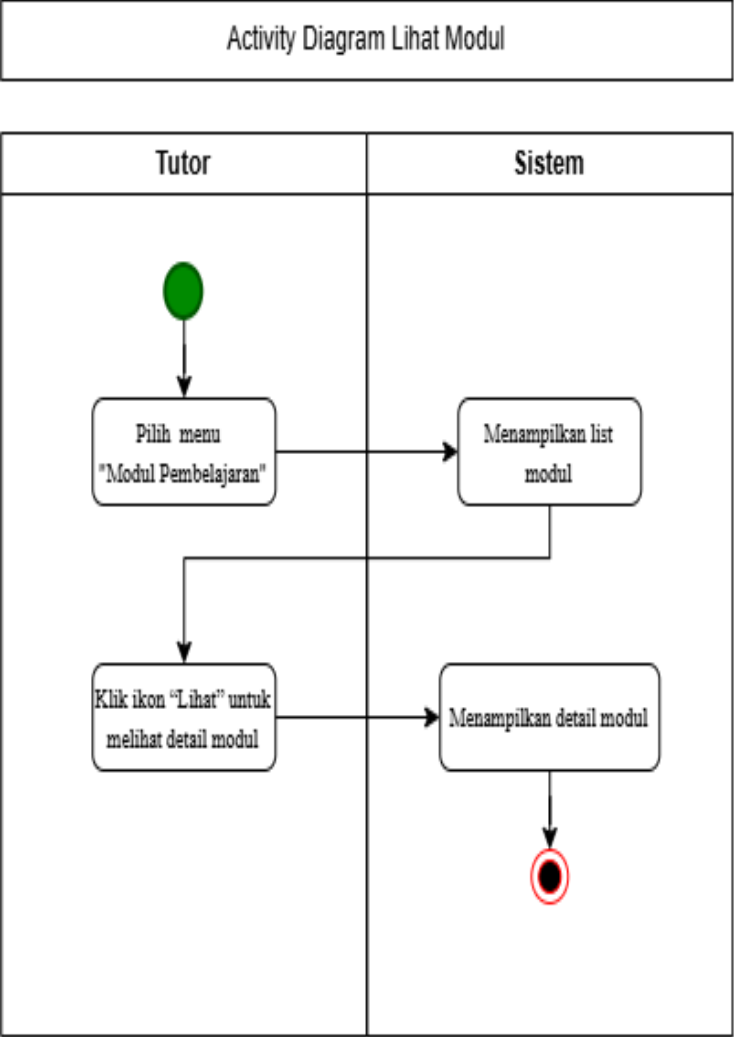
Gambar 6.17 Activity Diagram Tutor Melihat Modul Pembelajaran
