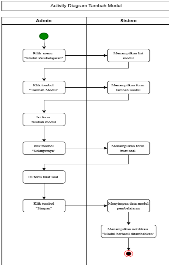
Gambar 6.2 Activity Diagram Menambah Modul Pembelajaran
