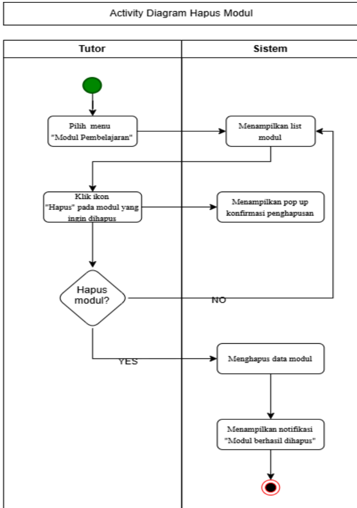
Gambar 6.16 Activity Diagram Tutor Menghapus Modul Pembelajaran
