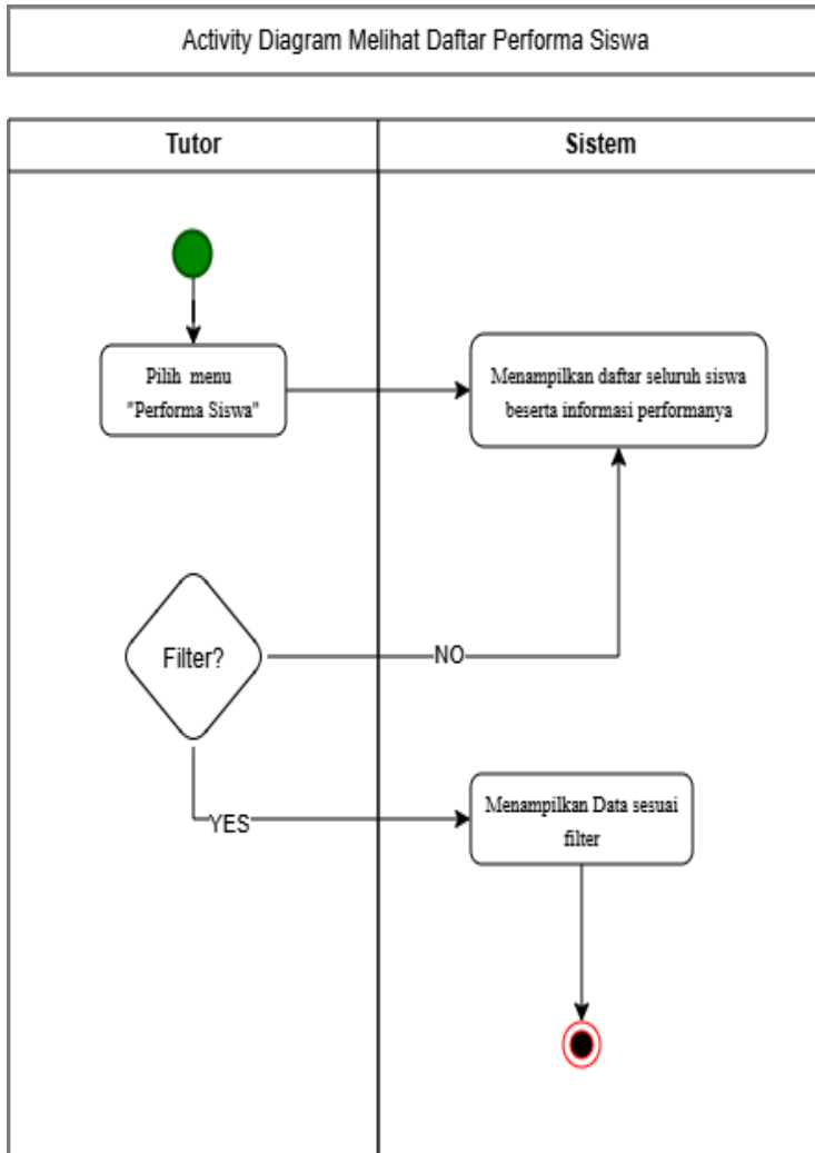
Gambar 6.18 Activity Diagram Tutor Melihat Daftar Performa Siswa
