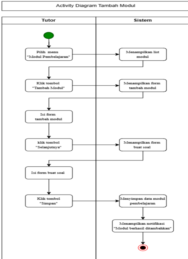
Gambar 6.15 Activity Diagram Tutor Menambah Modul Pembelajaran
