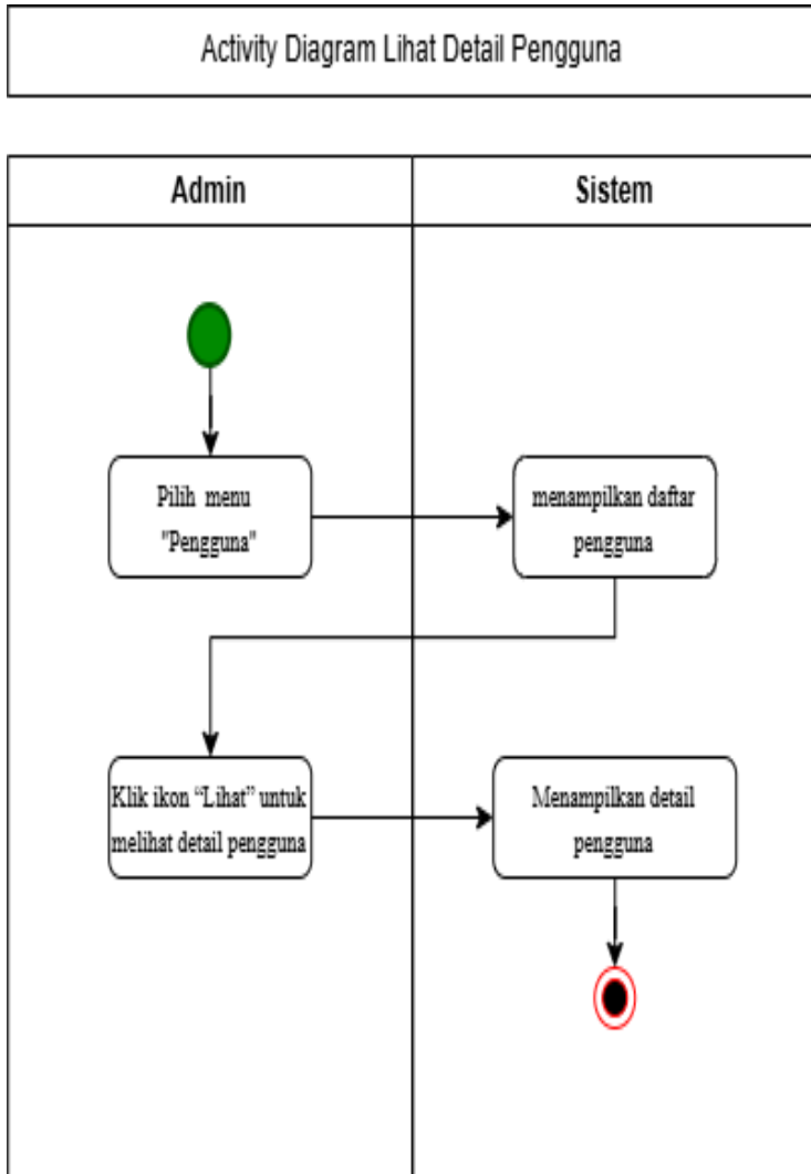
Gambar 6.13 Activity Diagram Melihat Detail Pengguna
