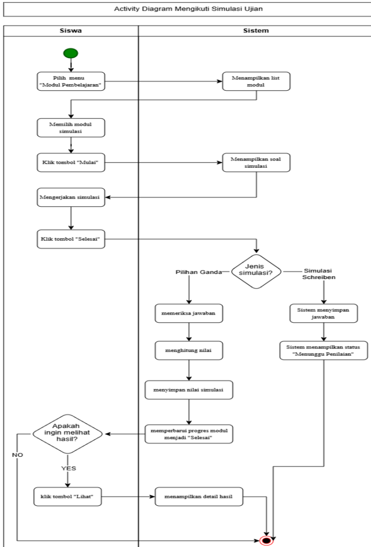
Gambar 6.22 Activity Diagram Siswa Mengikuti Simulasi Ujian
