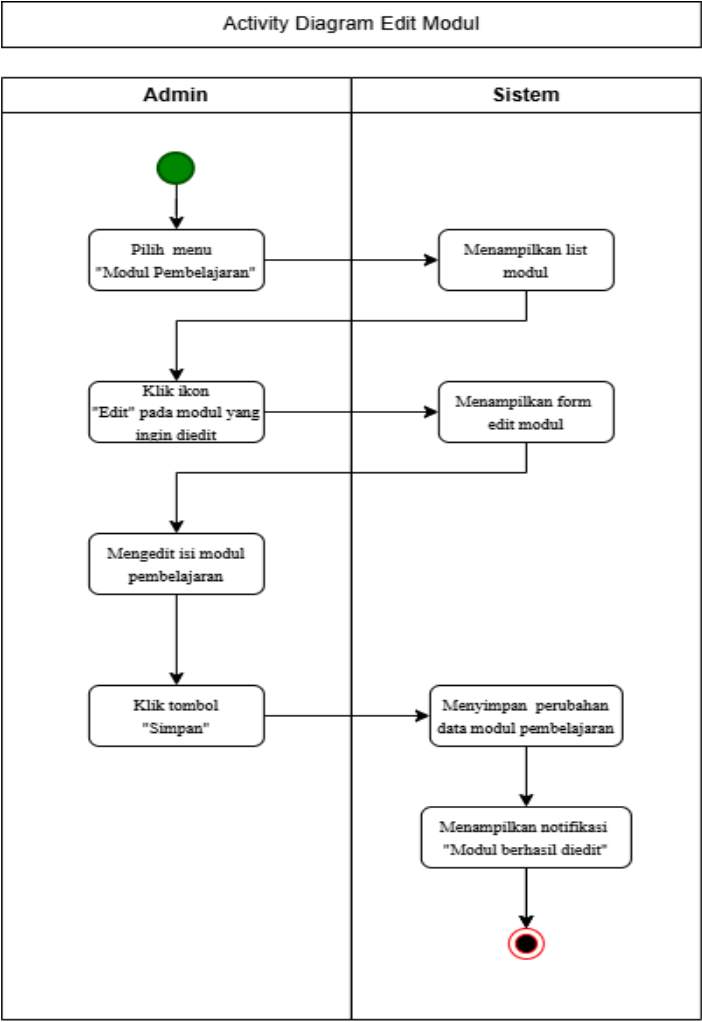
Gambar 6.3 Activity Diagram Mengedit Modul Pembelajaran
