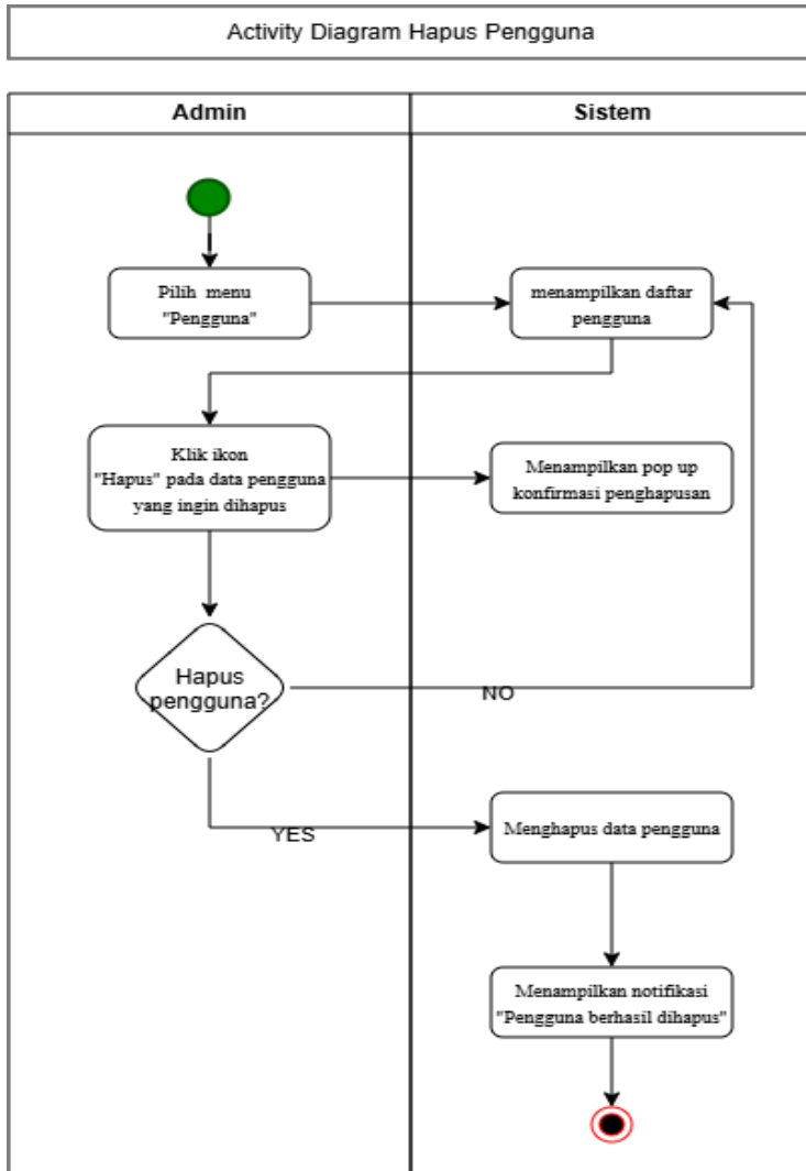
Gambar 6.12 Activity Diagram Menghapus Pengguna
