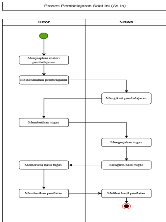
Gambar 4.1 BPMN Proses Pembelajaran Saat Ini (As-Is)
