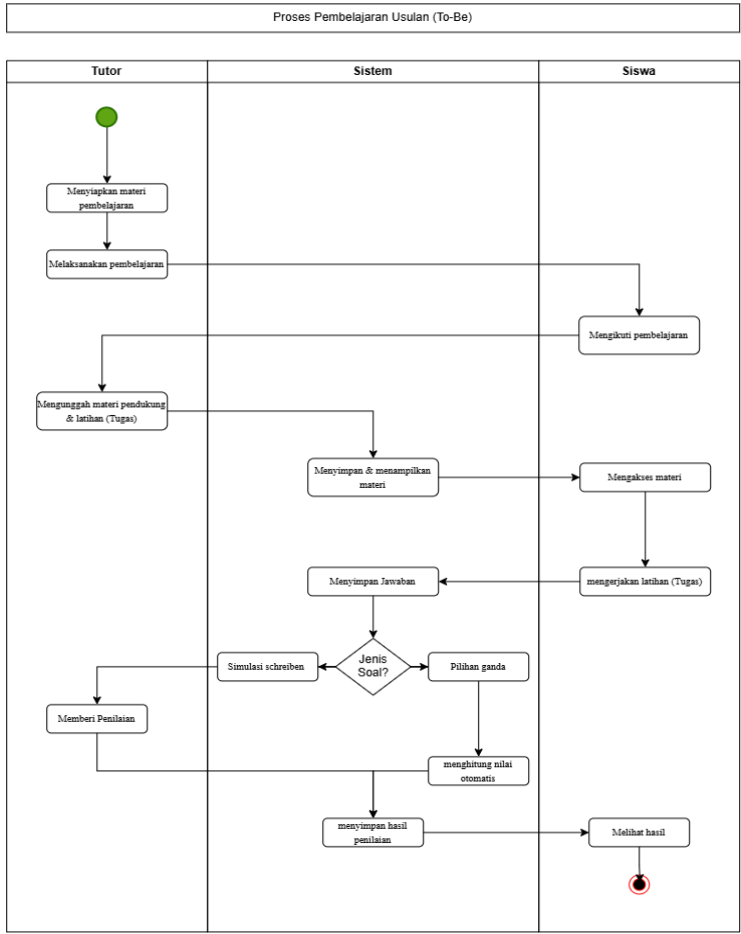
Gambar 4.2 BPMN Proses Pembelajaran Usulani (To-Be)
