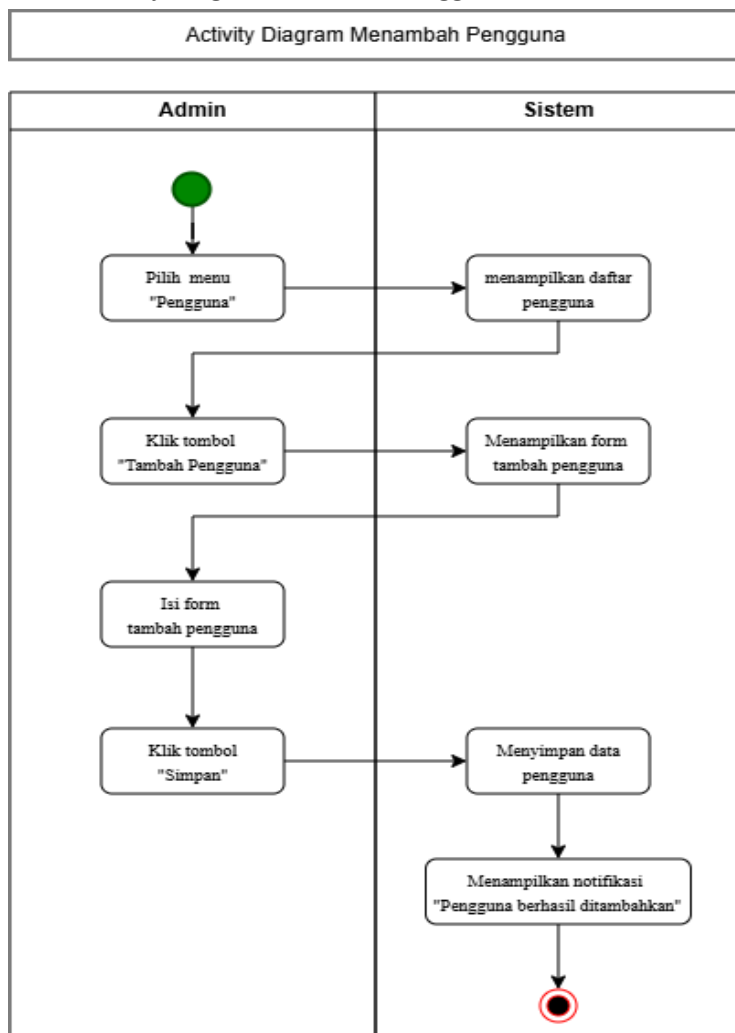
Gambar 6.10 Activity Diagram Menambah Pengguna
