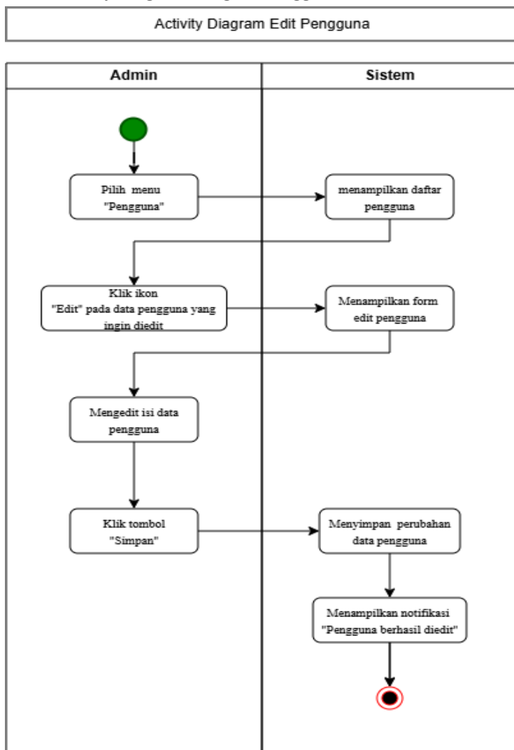
Gambar 6.11 Activity Diagram Mengedit Pengguna
